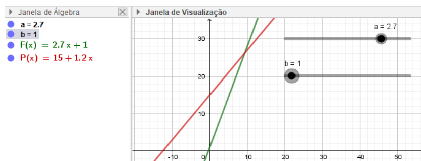
Figura 2: Gráfico (verde) da função polinomial de 1º grau com controles deslizantes
